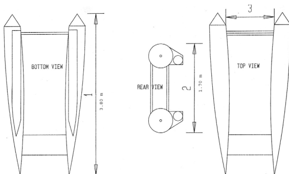
HULL DIAGRAM A:
